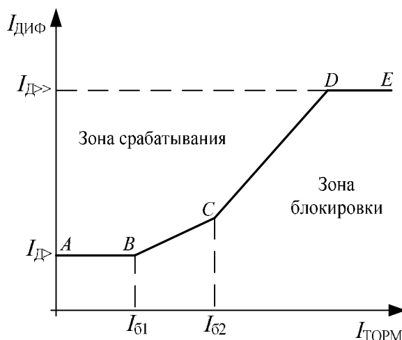
Рисунок 1 – тормозная характеристика.
